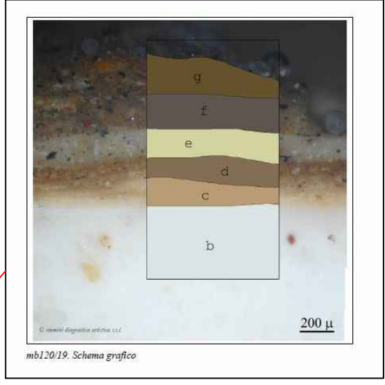
STRATIGRAFIA DELLE CORNICI
